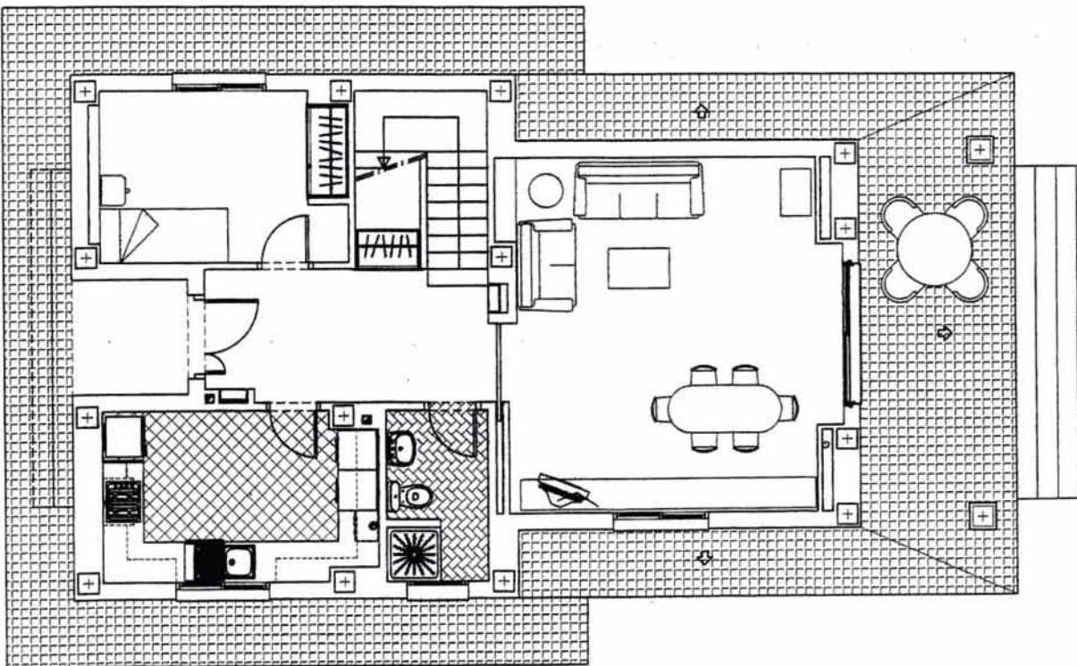
PLANTA BAJA
