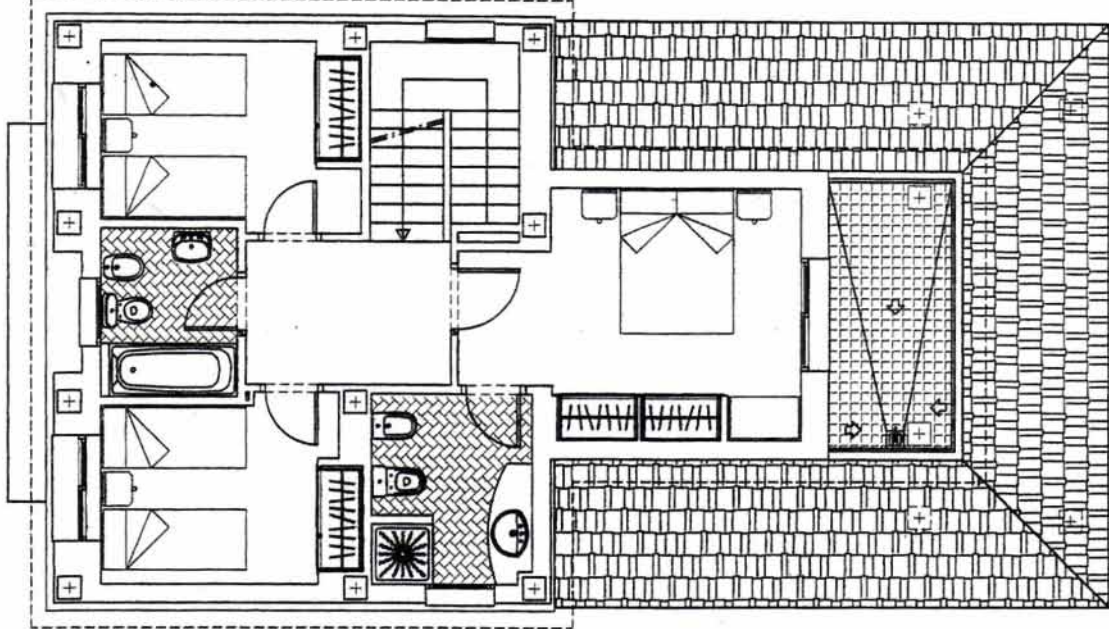
PLANTA PRIMERA
