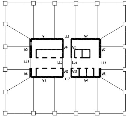
图 1 结构标准层平面布置简图
