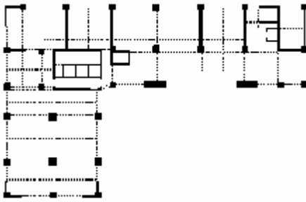
图 3a 裙房结构平面布置图
