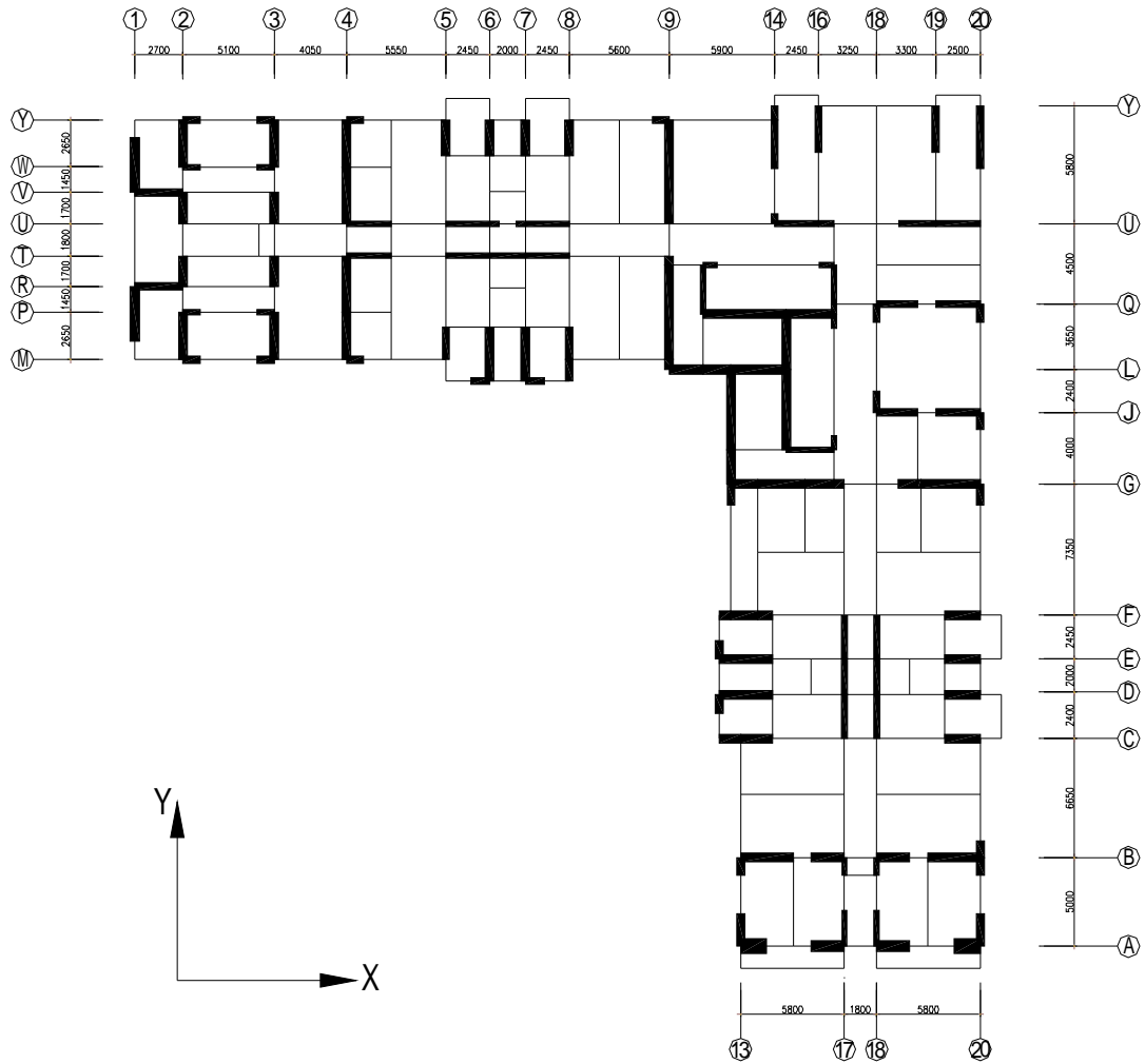
图2 结构标准层平面布置简图
