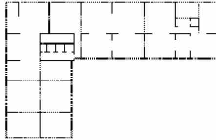
图 3b 标准层结构平面布置图
